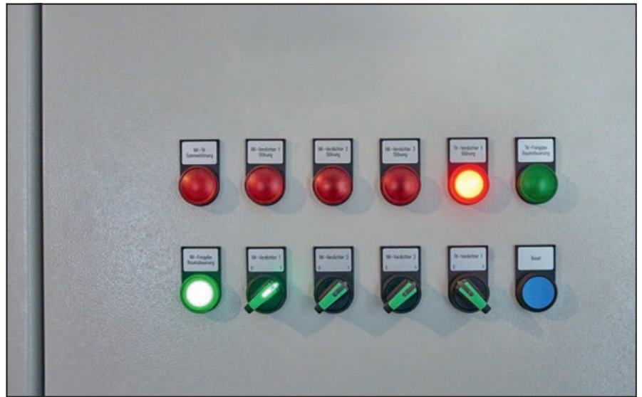
Robust und langlebig: Betriebsleuchten und Handschalter treffen auf eine im Hintergrund agierende digitale Regelung.
